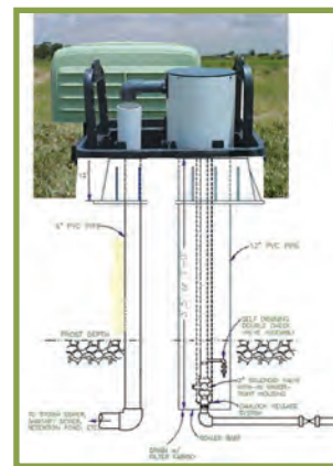
Dispositif Hydro-Guard MD S.M.A.R.T. MC HG-4
